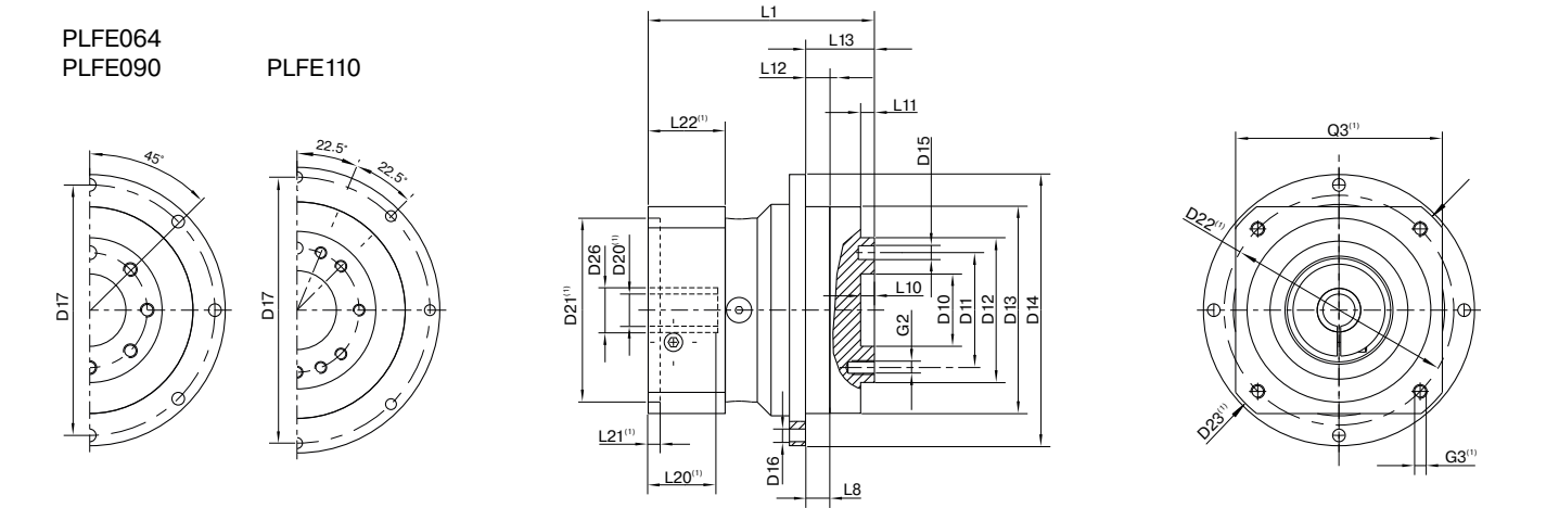
图示为带平键的 PLFE090 / 1 级 / 带有配合销孔的法兰输出轴 / 19 mm 锁紧系统 / 适配电机法兰 - 单一法兰 / B5 电机法兰类型 Drawing corresponds to a PLFE090 / 1-stage / flange output shaft with dowel hole / 19 mm clamping system / motor adaptation – one part / B5 flange type motor
