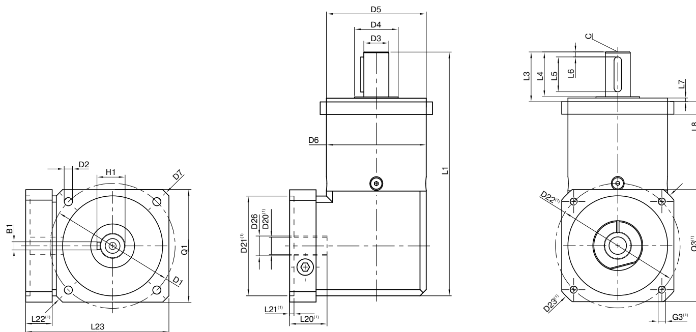
图示为带平键的 WPLQE080 / 1 级 / 附带平键的输出轴 / 19 mm 锁紧系统 / 适配电机法兰 - 2 件式 - 正方形通用法兰 / B5 电机法兰类型
