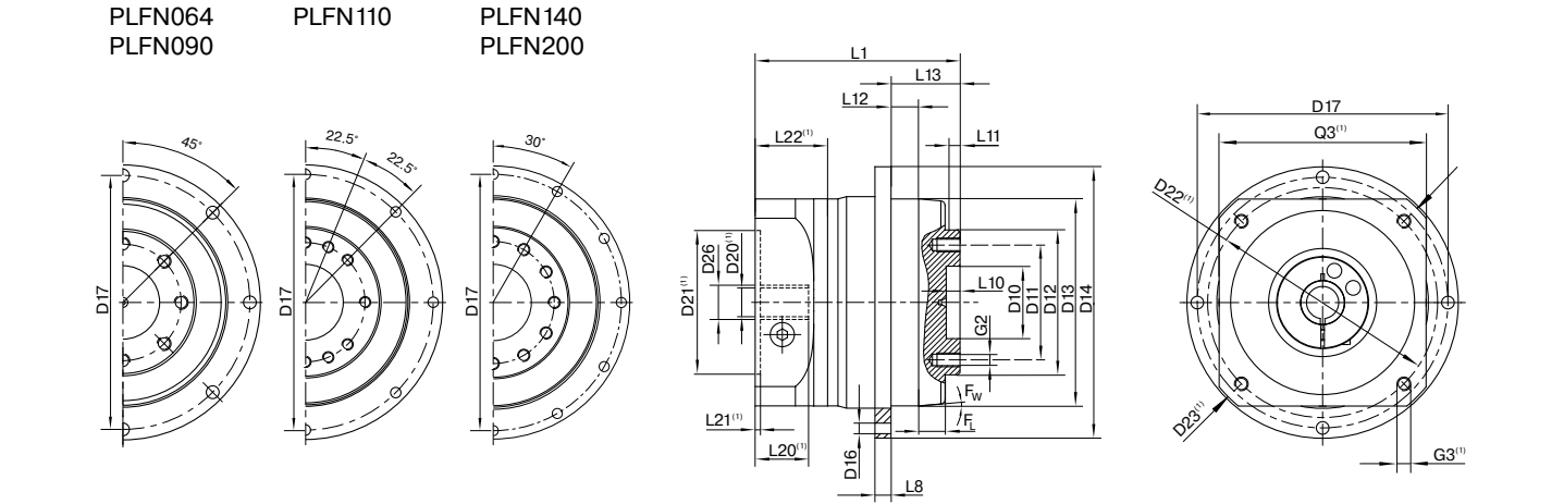
图示为带平键的 PLFN090 / 1 级 / 法兰输出轴 / 19 mm 锁紧系统 / 适配电机法兰 – 2 件式 – 圆形通用法兰 / B5 电机法兰类型 Drawing corresponds to a PLFN090 / 1-stage / flange output shaft / 19 mm clamping system / motor adaptation – 2-part – round universal flange / B5 flange type motor (1) 具体尺寸视电机/减速机法兰而定。可以在 www.neugart.com 下 Tec Data Finder。中针对每个电机适配电机特有的输入法兰几何尺寸。 (1) The dimensions vary with the motor/gearbox flange. The input flange dimensions can be retrieved for each specific motor in Tec Data Finder at www.neugart.com
